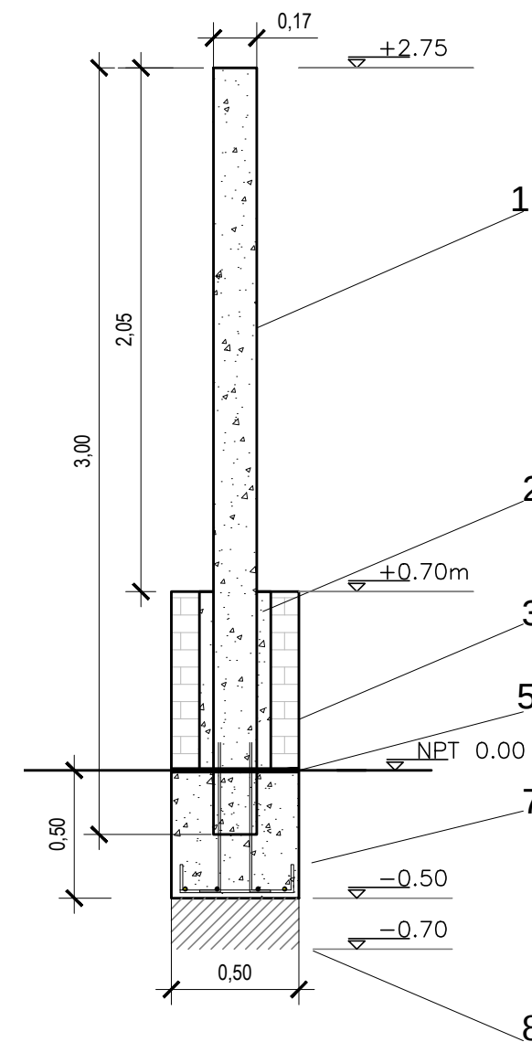
CORTE A-A POR COLUMNA
